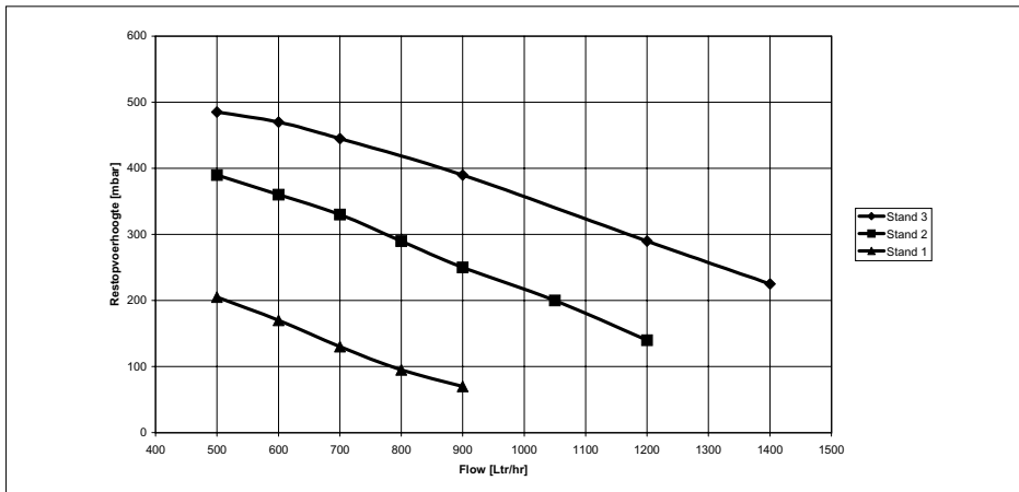
Afb 15. Grafiek restopvoerhoogte t.b.v. de c.v.-installatie
