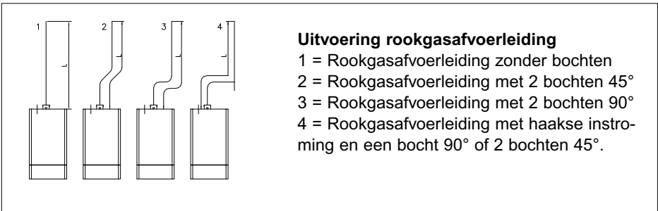
Afb 13. Standaardsituaties 'open uitvoering'
