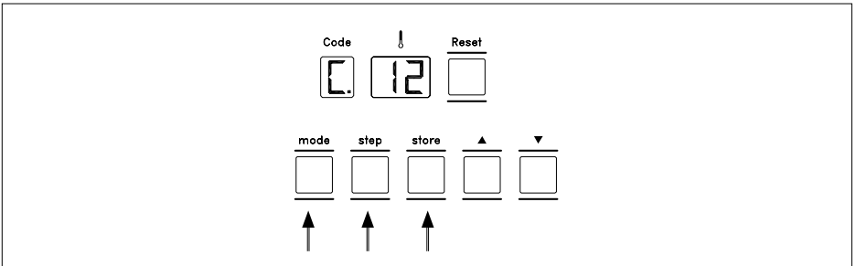
Afb 10. Toegangsbevestiging servicecode 00W3H7900024
