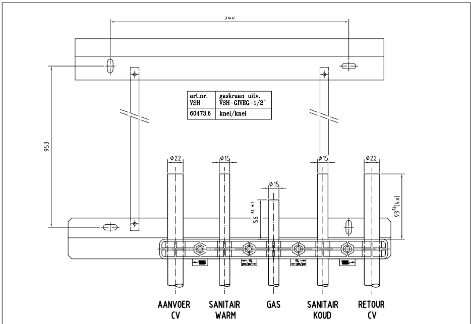
Afb 12. Montagebeugel (optie)
