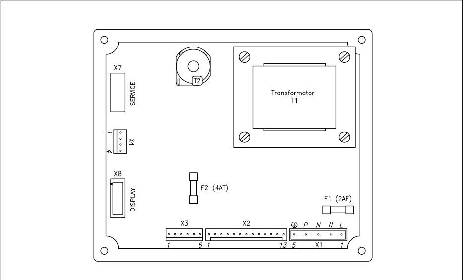
Afb 20. Beveiligingsautomaat Gasmodul 00W4H7900018
