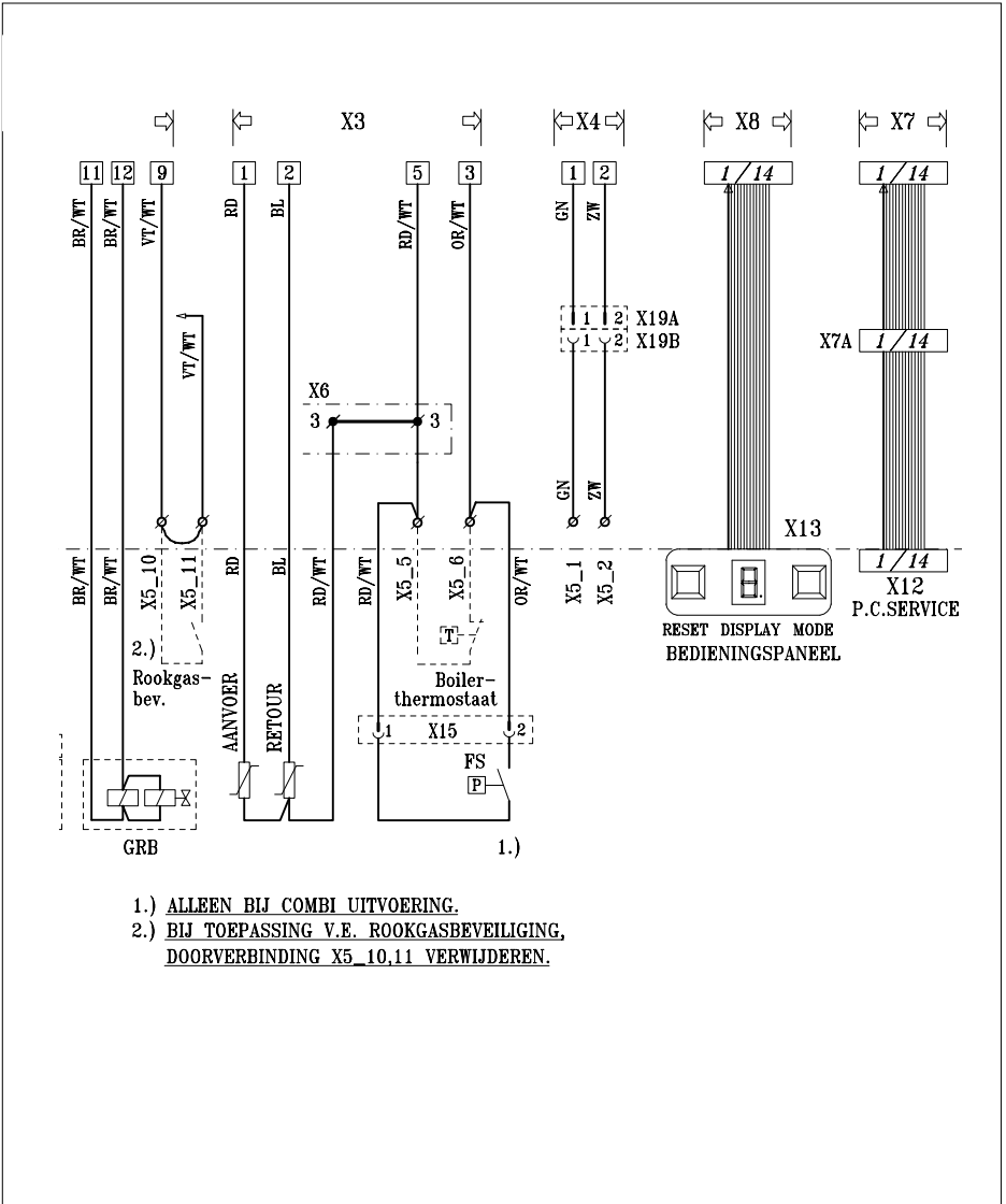
Afb 22. Elektrisch schema deel 2 00W3HSC02273
