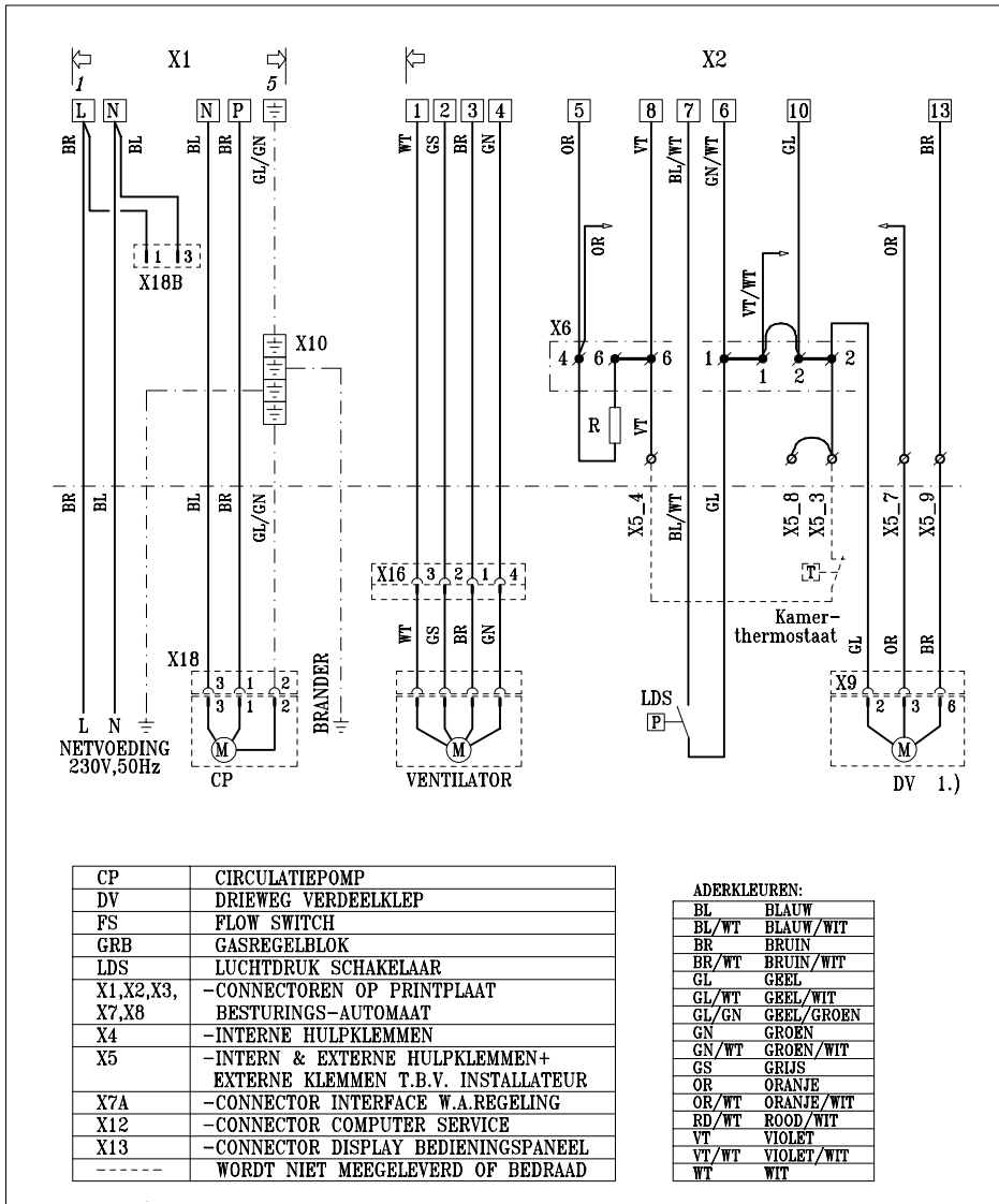
Afb 21. Elektrisch schema deel 1
