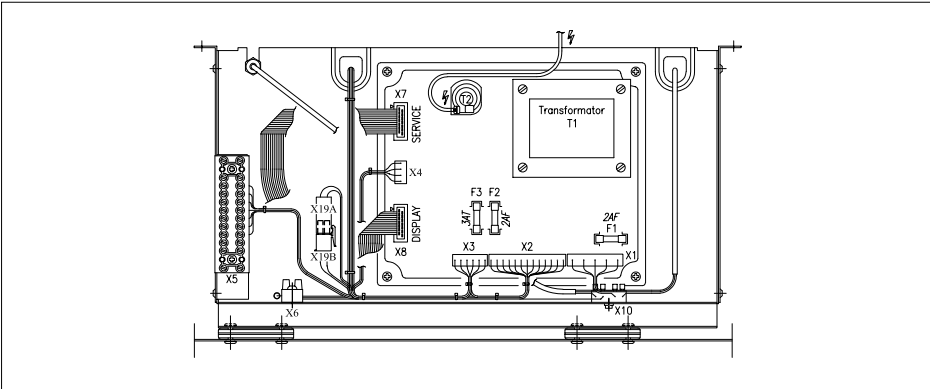
Afb 25. Overzicht instrumentenkast 00W3H7900036
