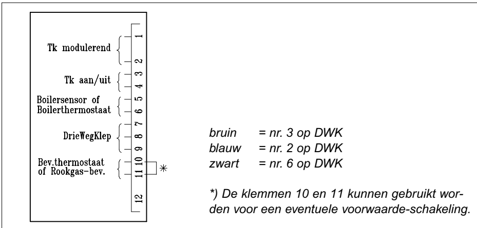
Afb 19. Aansluitingen op de klemmenstrook
