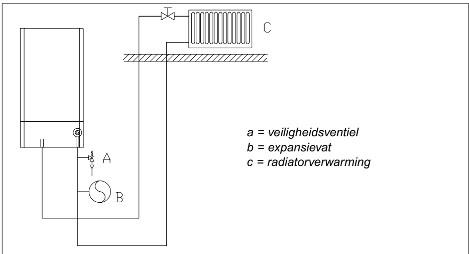
Afb 16. Veiligheidsvoorzieningen bij W21/28 ECO
